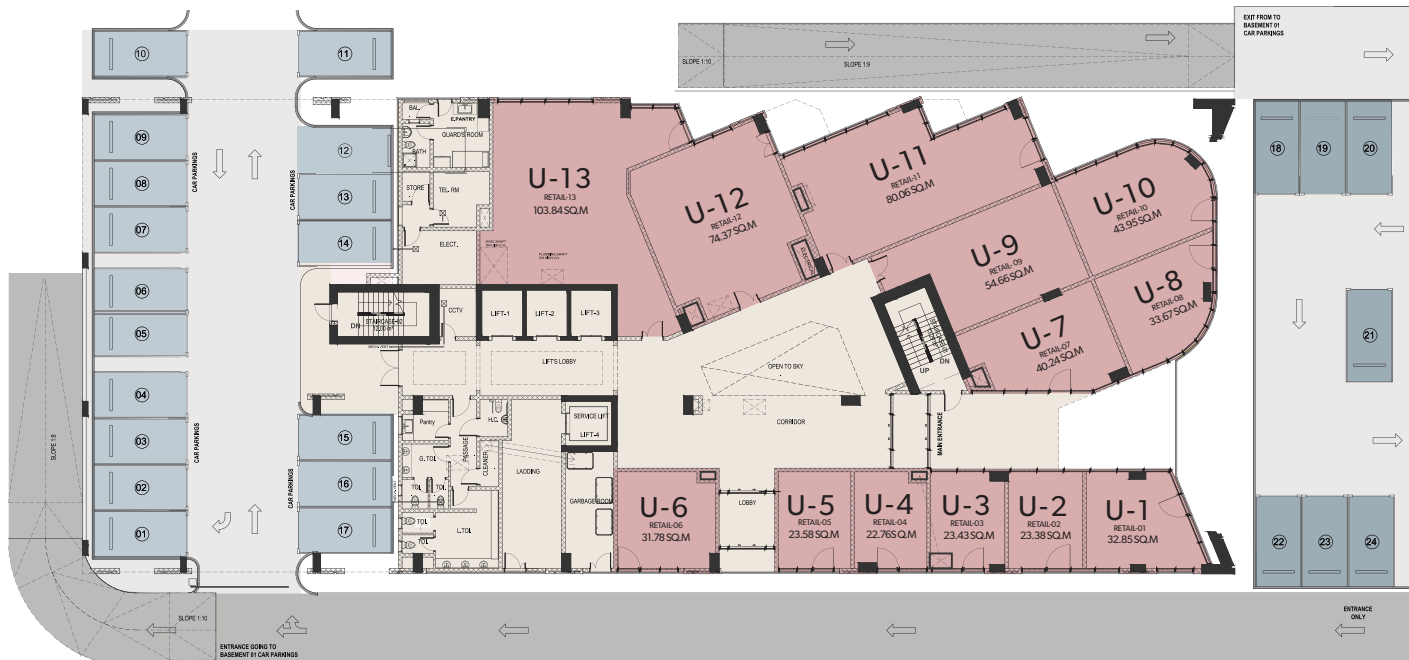
مخطط الطابق الأرضي Ground Floor Plan
