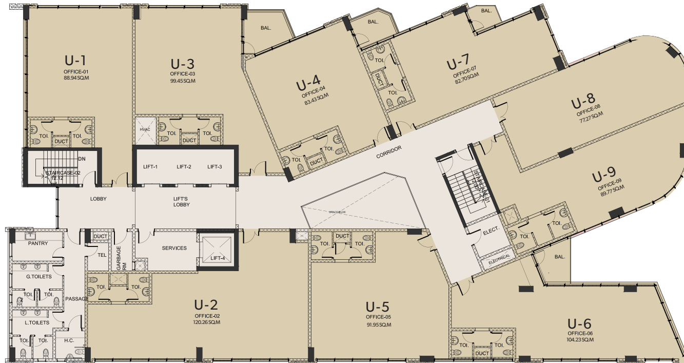
مخطط الطابق السادس Sixth Floor Plan
