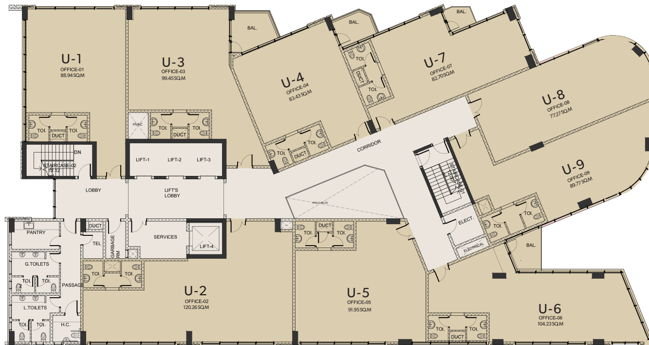
مخطط الطابق الرابع Forth Floor Plan
